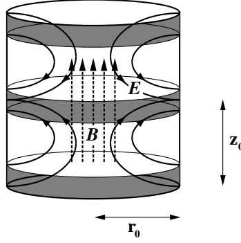
Figure 4.32: Configurazione dei campi elettrico e magnetico in una Penning trap .
