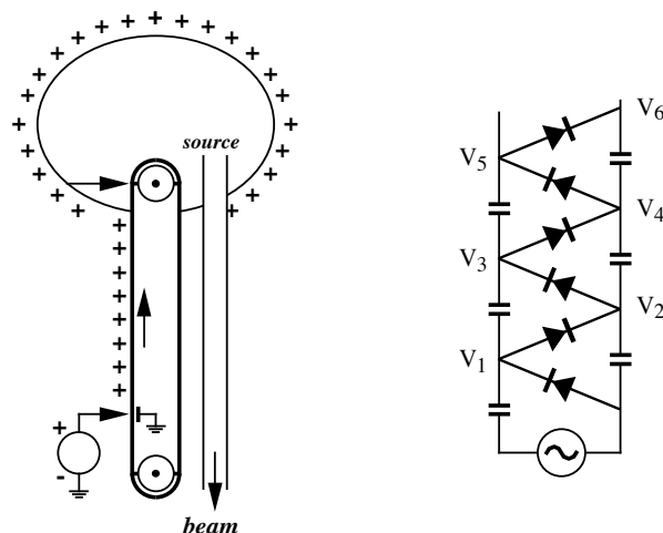
Figure 1.16: Principio di funzionamento degli acceleratori elettrostatici
