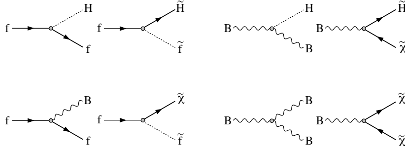
Figure 4.37: Accoppiamenti di particelle e campi e dei corrispondenti super-partner. Fermione: linea continua, bosone scalare: linea tratteggiata, bosone di gauge: linea ondulata.
