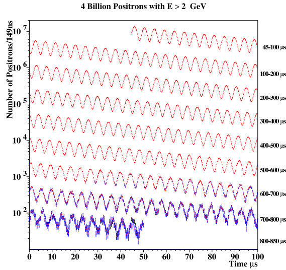
Figure 4.36: Conteggio di e^+ in funzione del tempo per la misura dell'anomalia del \mu^+ (G.W.Bennett et al. , Physical Review D73, 072003, 2006).
