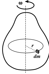
Figure 4.31: Momento magnetico e momento angolare di un corpo rigido in rotazione.
