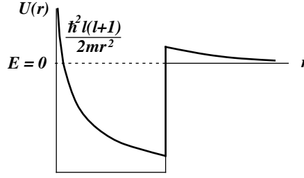
Figure 4.14: Buca di potenziale e potenziale centrifugo
