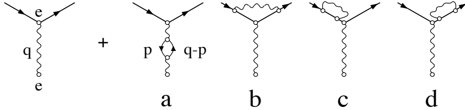
Figure 4.22: Grafici al primo ordine, \mathcal{O}(e^2) , e al secondo ordine, \mathcal{O}(e^4) , dell'interazione elettromagnetica
