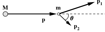
Figure 4.8: Collisione tra una particella di massa M e impulso \vec{p} e una particella di massa m in quiete
