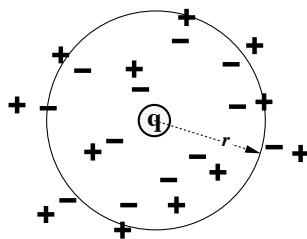
Figure 4.23: Polarizzazione del vuoto
