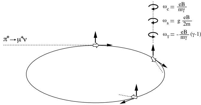
Figure 4.34: Moto di rivoluzione del muone e di precessione dello spin.
