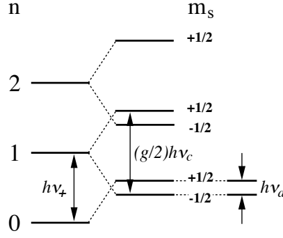
Figure 4.33: Livelli energetici dell'elettrone in una Penning trap .
