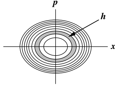
Figure 1.3: Quantizzazione dell'oscillatore armonico
