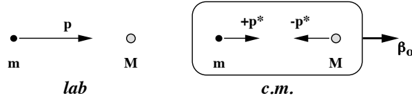
Figure 4.7: Riferimenti del laboratorio e del centro di massa
