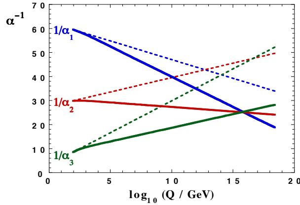
Figure 4.38: Costanti di accoppiamento dei campi di gauge, 1/\alpha_i , in funzione della scala di energia di interazione. Modello Standard: linee tratteggiate, MSSM: linee continue.
