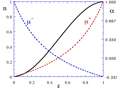
Figure 4.35: Numero di elettroni n(\epsilon) e asimmetria \alpha(\epsilon) nel riferimento del muone.
