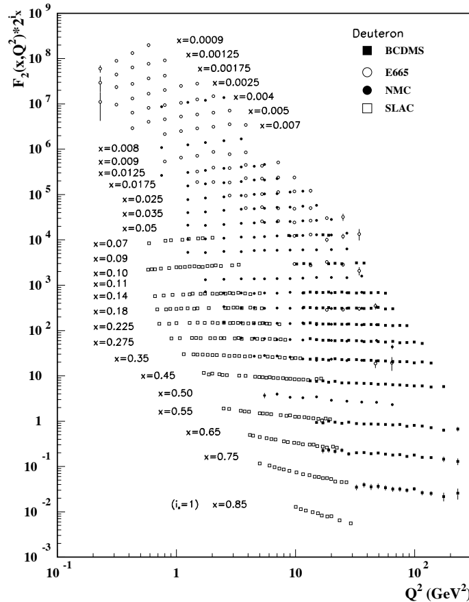
Figure 3.63: Funzione di struttura F_2(x, Q^2) misurata con deuterio (S. Eidelman et al., Phys. Lett. B592, 1, 2004) nota : \times 2 per x = 0.85 , \times 4 per x = 0.75, \dots
