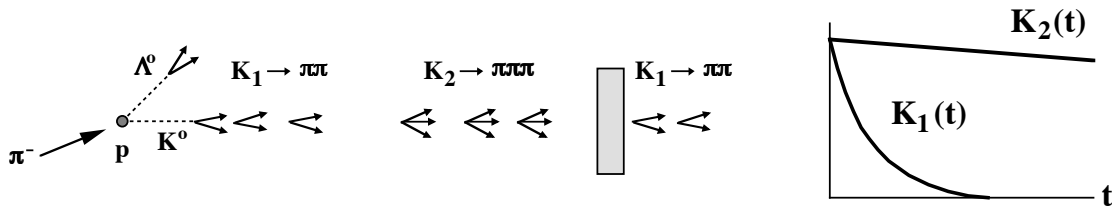
Figure 3.28: Decadimento e rigenerazione di un fascio di mesoni K^0
