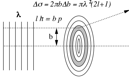
Figure 1.59: Diffusione da un disco assorbente
